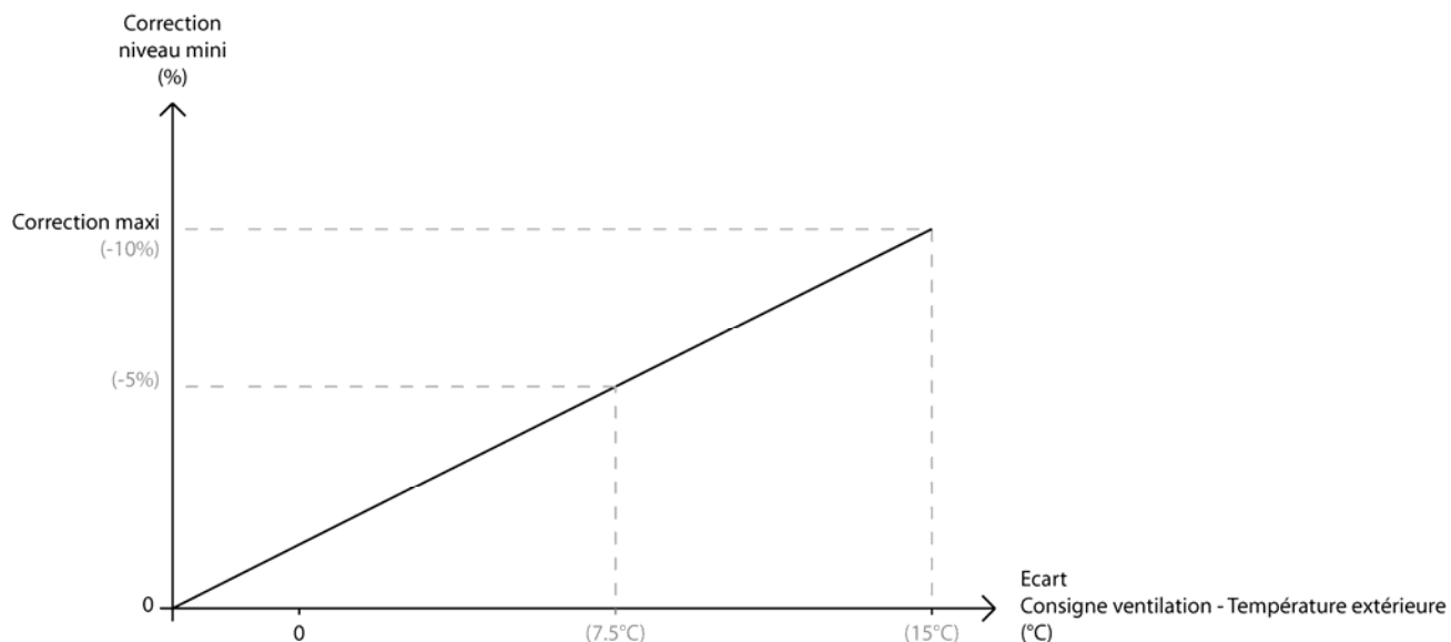
Influence de la température extérieure sur le mini treuil
