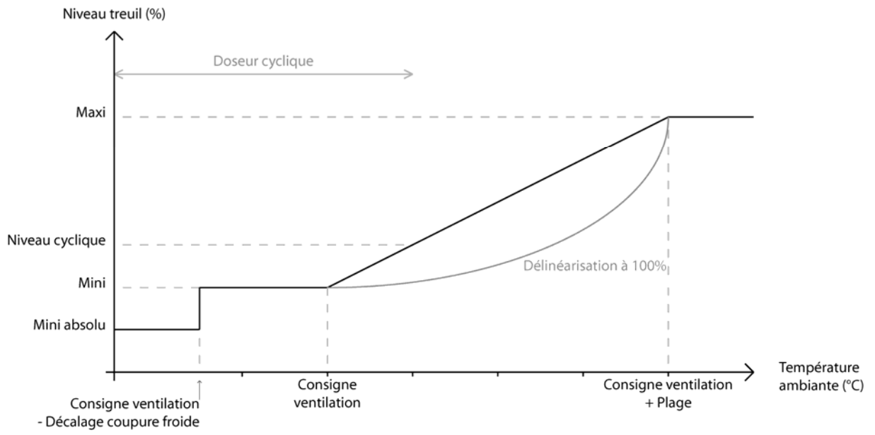
Mini Fixe + Coupure Froide
