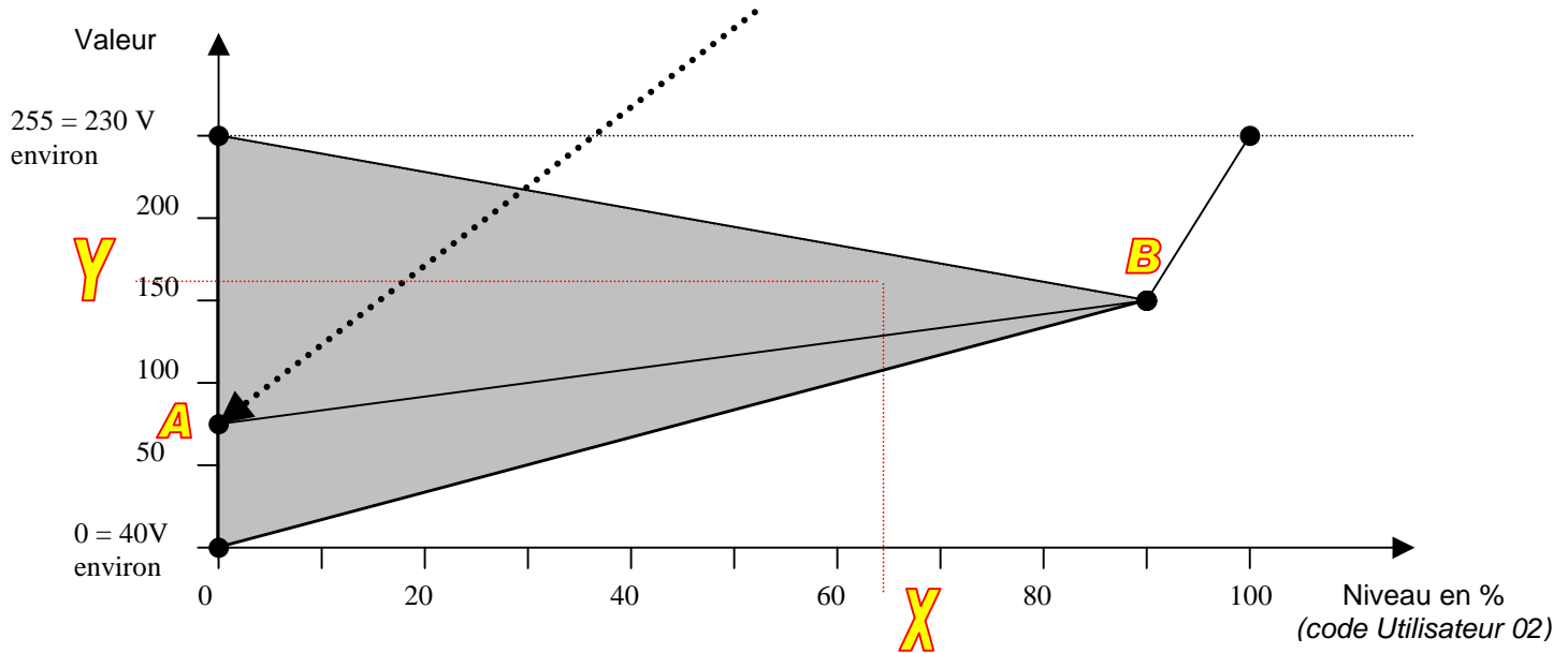
Réglage du ralenti effectué en partie Installateur (code Installateur 20)
