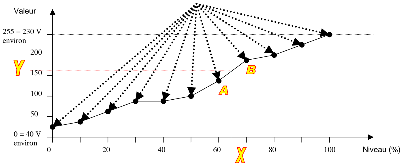
Réglages effectués en partie Installateur (codes 20 à 30)
